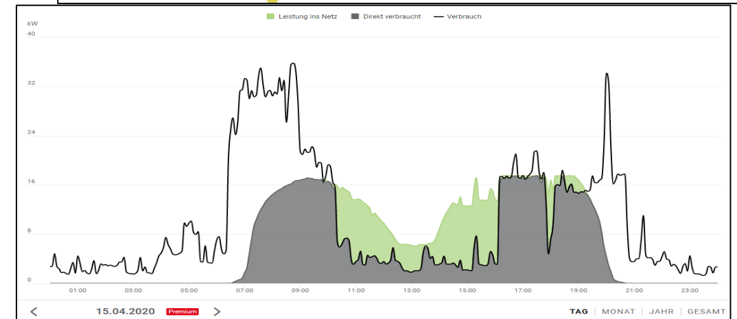
Eigenverbrauch Milchviehbetrieb in Irland
