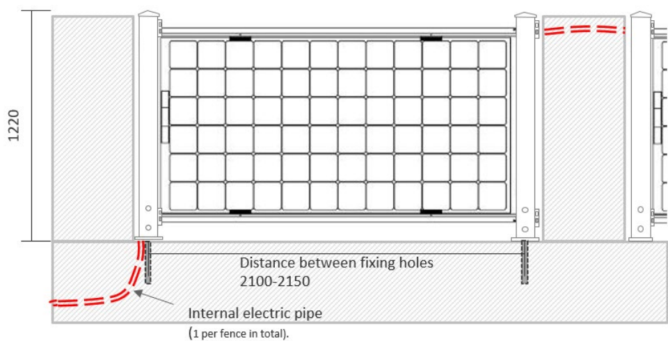
Aufmauer-Montage
